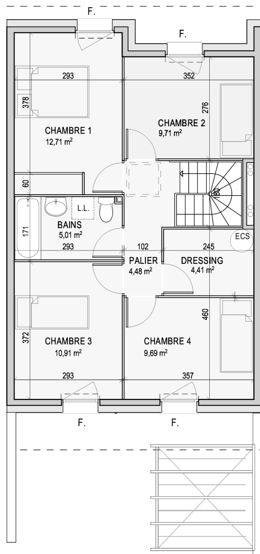
Plan de l'étage 1/100
